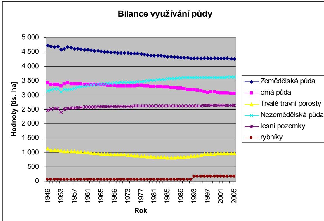
Graf 4: Bilance využívání půdy
