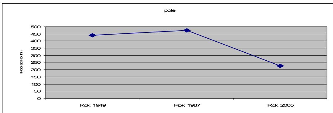
Graf 13: plocha polí
