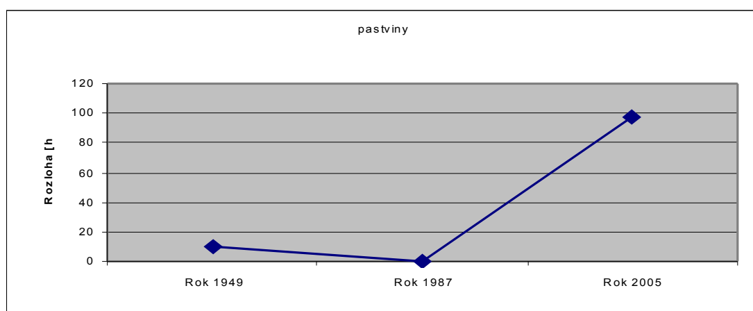
Graf 11: plocha pastvin
