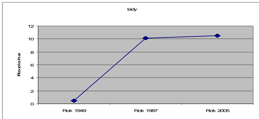
Graf 12: plocha lad
