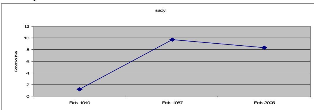
Graf 17: plocha sadů
