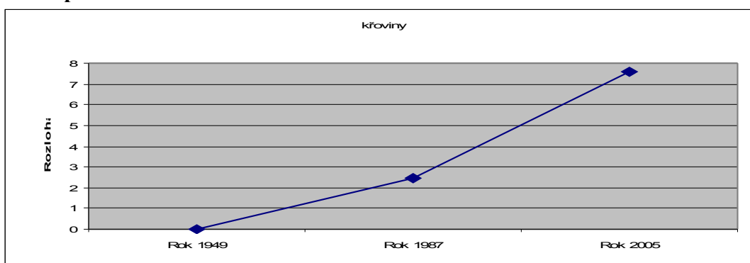
Graf 14: plocha křovin
