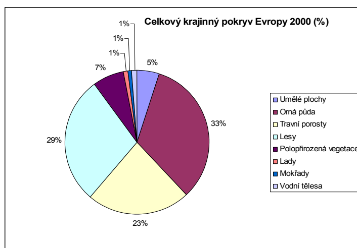
Graf 5: Celkový krajinný pokryv (Total land cover) Evropy (Anonymous, 2006):
